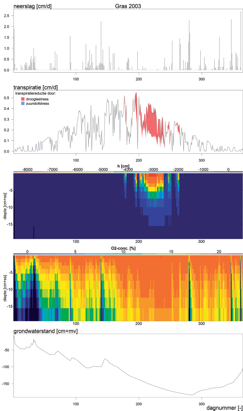
Afbeelding 4: Dagelijkse neerslag (boven); potentiële transpiratie, actuele transpiratie (tweede figuur), en transpiratiereductie veroorzaakt door droogtestress of zuurstofstress (tweede figuur, respectievelijk bovenste lijn, onderste lijn, rood en blauw vlak); drukhoogteprofiel in de wortelzone (derde figuur), zuurstofprofiel in de wortelzone (vierde figuur) en grondwaterstandsverloop (onder), voor gras (worteldiepte 20 cm) op zwak-lemig zand ('casus Ruurlo') en het droge jaar 2003.
